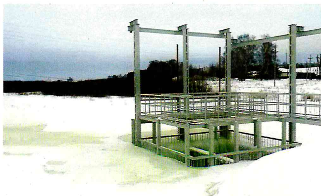
ГТС в д. Холкина после капитального ремонта.
